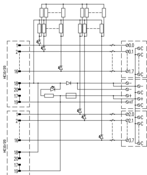
Kopplingsbilden motsvarar utförandet med LED
