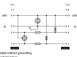
Komplettsmodul
