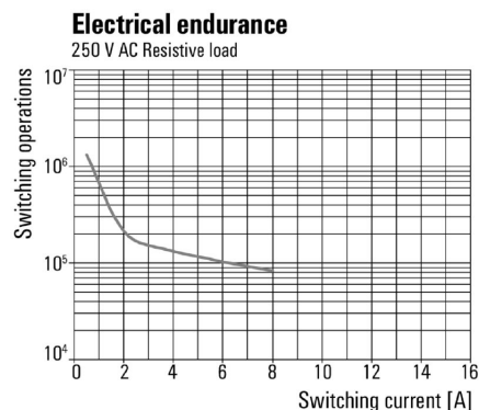
Elektrisk livslängd 250 V AC ohmsk last
