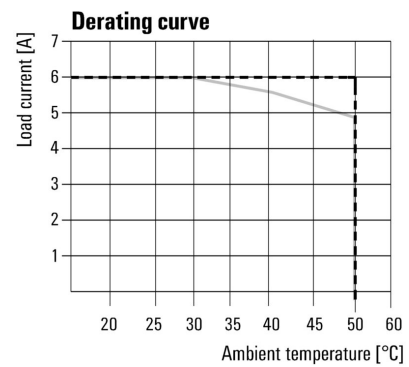
Deratingkurva
