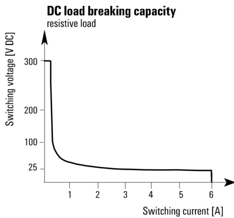
DC-lastgränskurva
