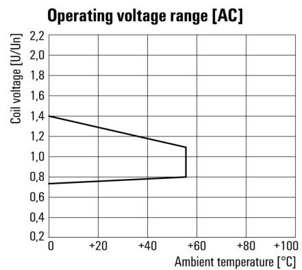
AC-driftspänningsområde
