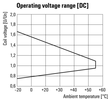
DC-driftspänningsområde
