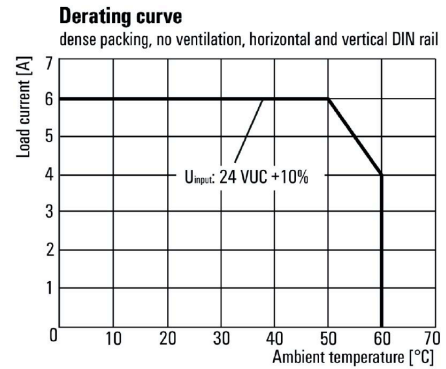
Deratingkurva
