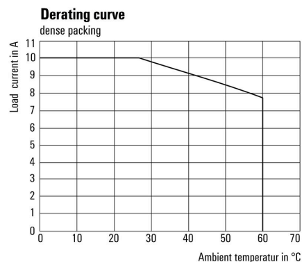
Deratingkurva
