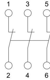
Trefasigt anti-open-principkopplingsschema
