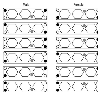
Kodningsschema
