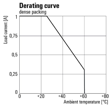
Deratingkurva
