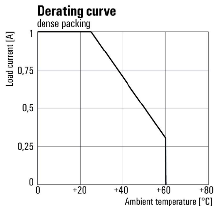
Deratingkurva
