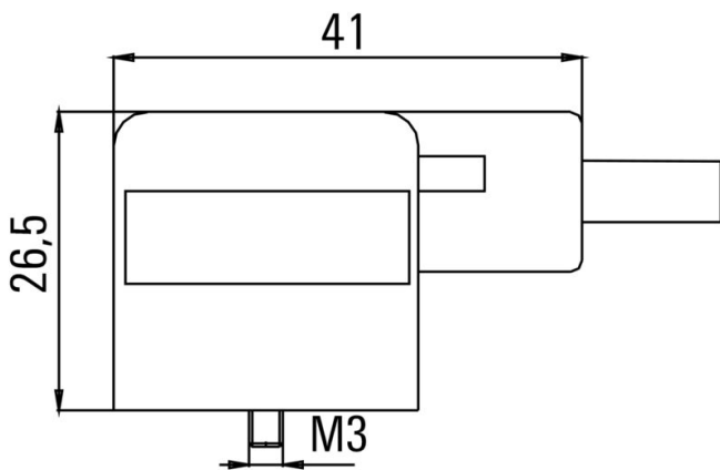
Габаритный чертеж
