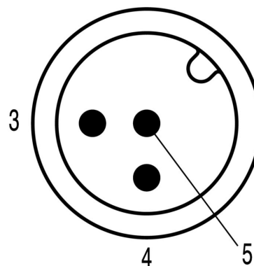
Схема контактов
