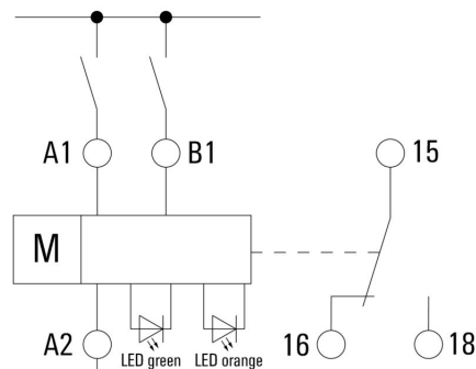
Пример электромонтажа
