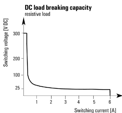
Кривая предельной нагрузки пост. тока
