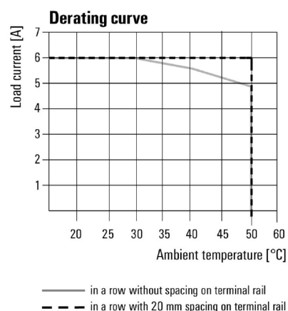
Кривая ухудшения параметров
