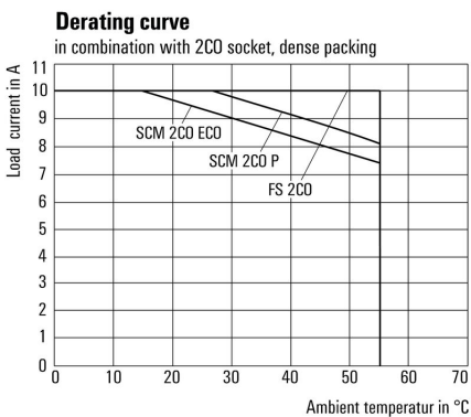
Кривая ухудшения параметров Реле в сочетании с основанием
