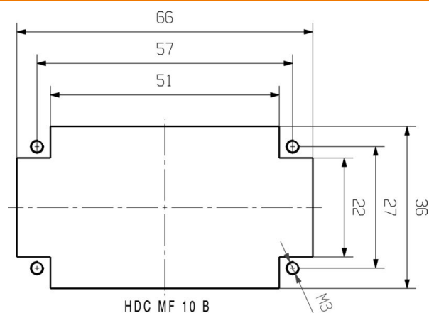
монтажный вырез
