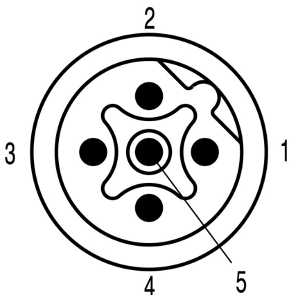
Схема контактов
