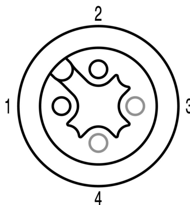
Схема контактов
