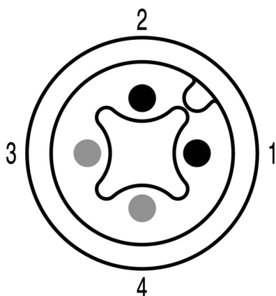
Схема контактов
