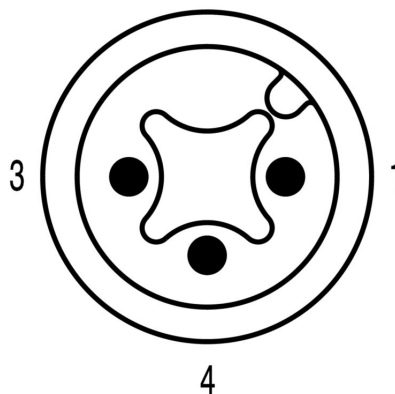
Схема соединений
