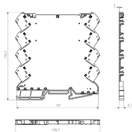
Габаритный чертеж
