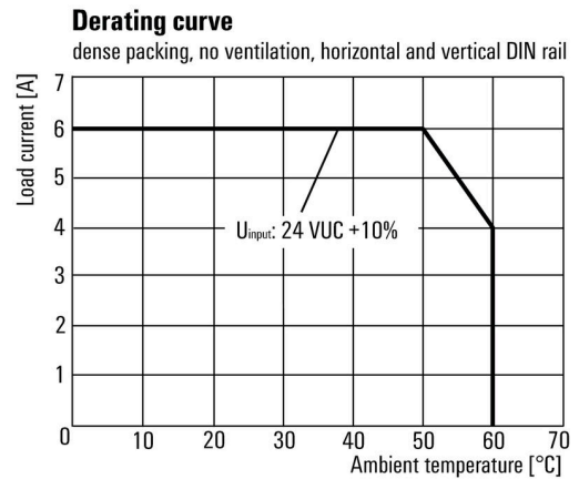
Кривая ухудшения параметров
