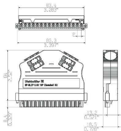
Габаритный чертеж
