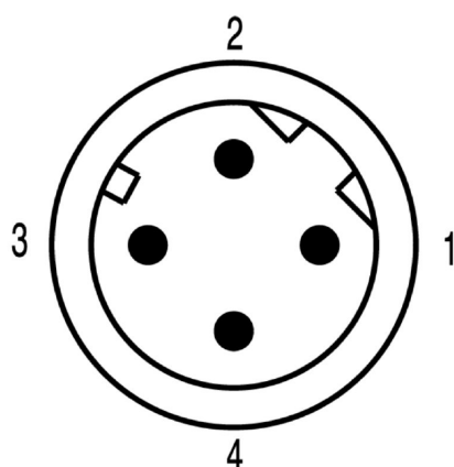
Схема контактов
