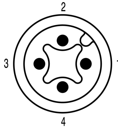
Схема контактов
