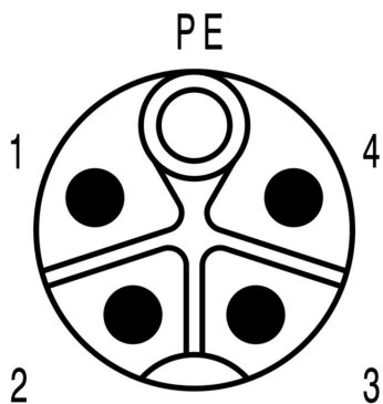
Схема контактов
