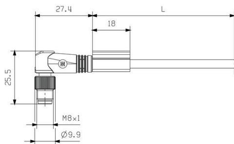
Габаритный чертеж
