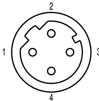
Схема контактов
