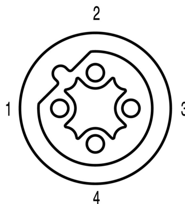
Схема контактов
