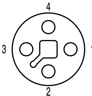
Схема контактов
