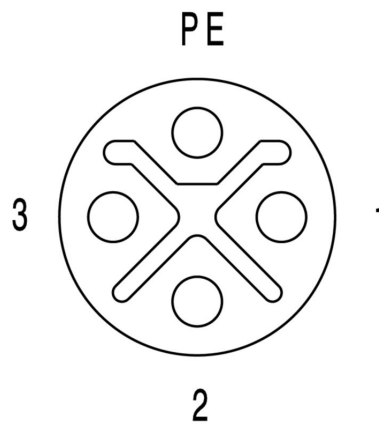
Схема контактов
