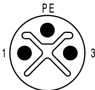
Схема контактов
