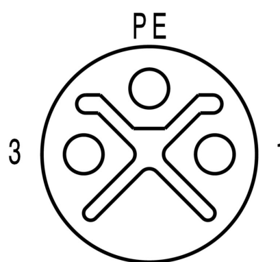
Схема контактов
