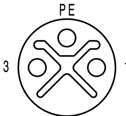
Схема контактов
