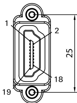
Габаритный чертеж
