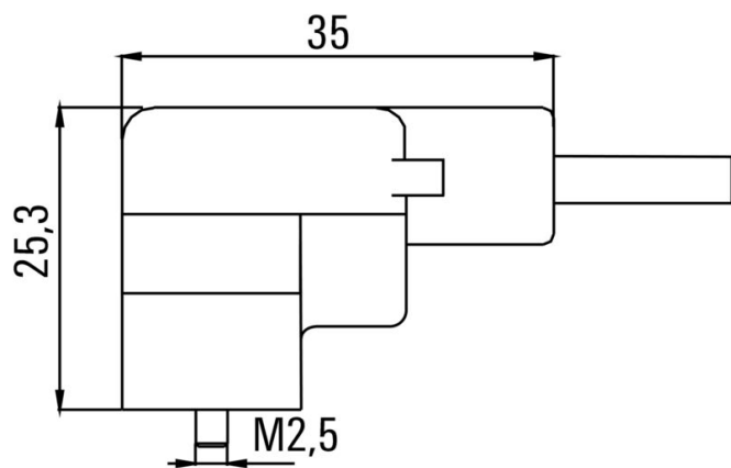
Габаритный чертёж
