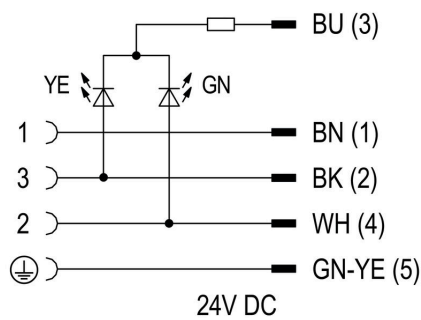
Схема соединений
