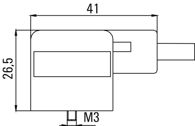
Габаритный чертеж
