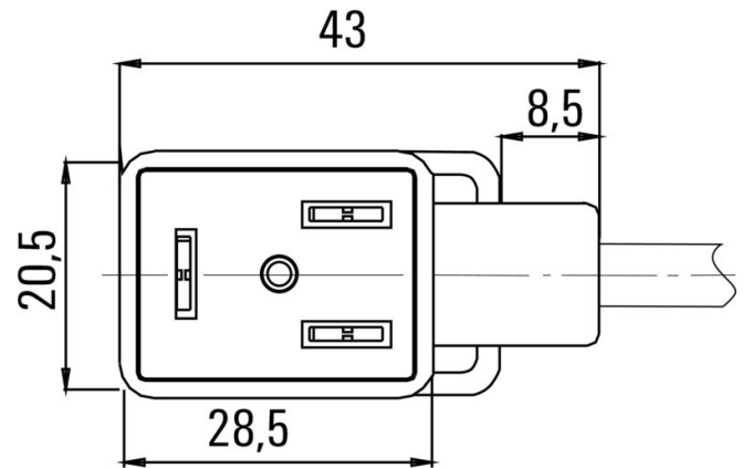
Схема контактов
