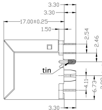
Габаритный чертёж
