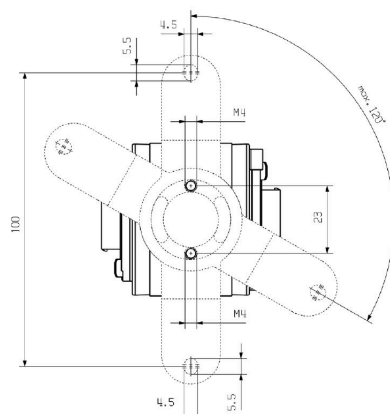
Габаритный чертеж
