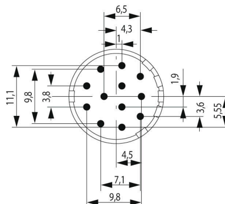
Габаритный чертеж
