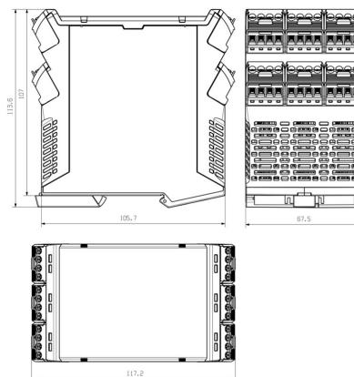
Габаритный чертёж
