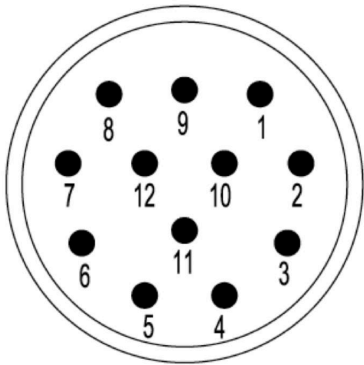
Развод контактов
