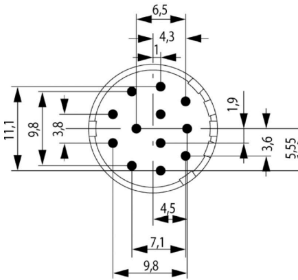
Габаритный чертеж
