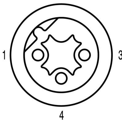
Socket
