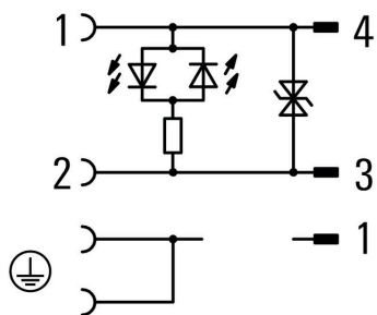
Схема соединений
