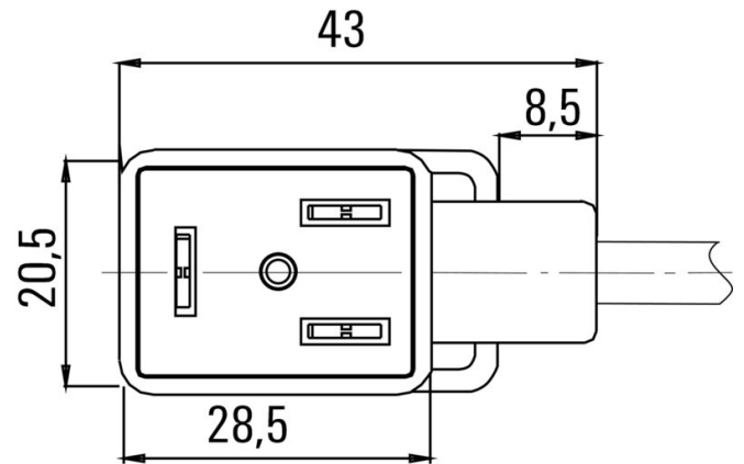
Schemat biegunów
