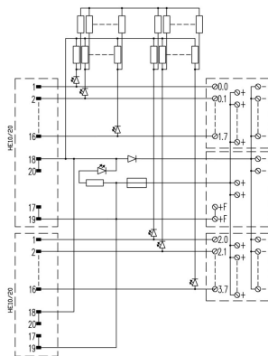
Schemat dotyczy wersji z ledami
