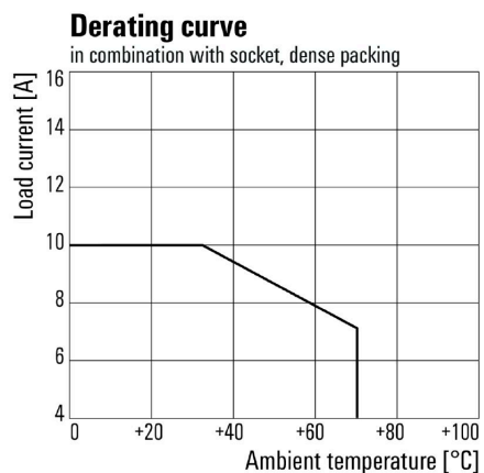
Krzywa obciążalności prądowej Przełącznik połączony z podstawką
