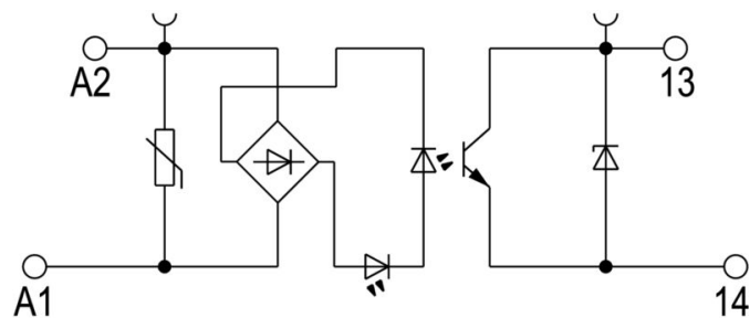
Schaltssymbol
